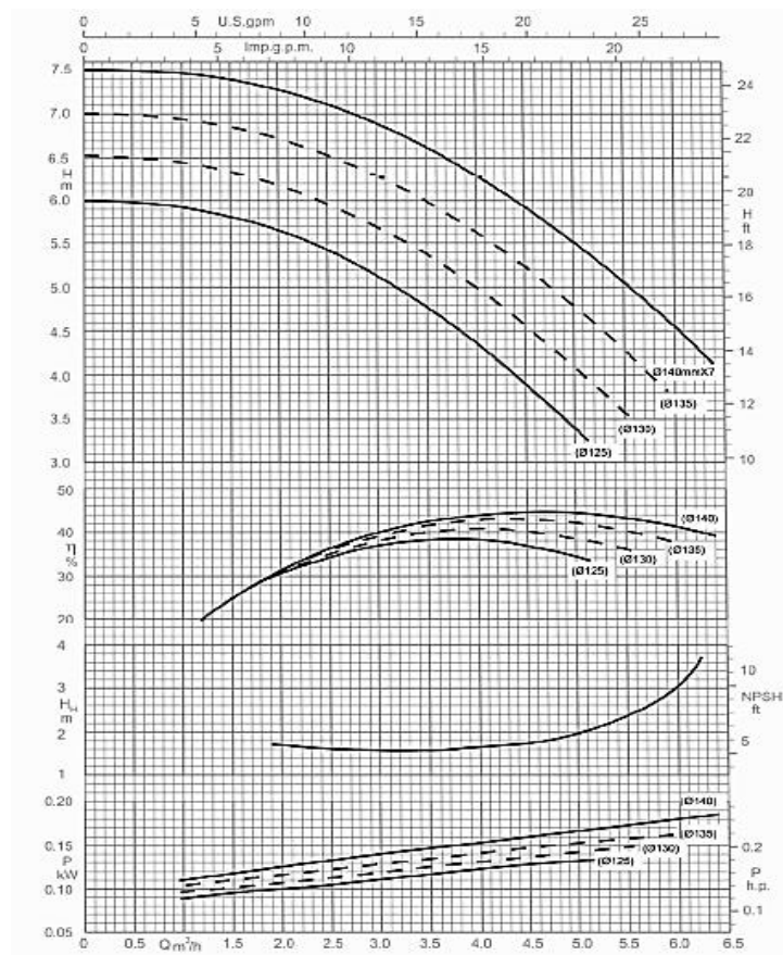
دور موتور ۱۴۵۰ منحنی یک طبقه
