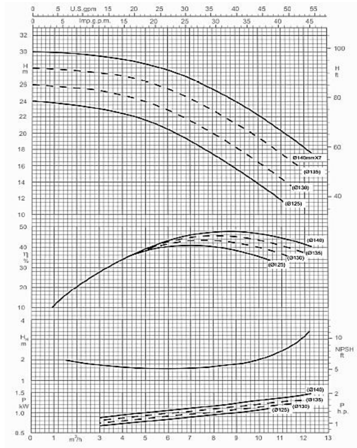
دور موتور ۲۹۰۰ منحنی یک طبقه
